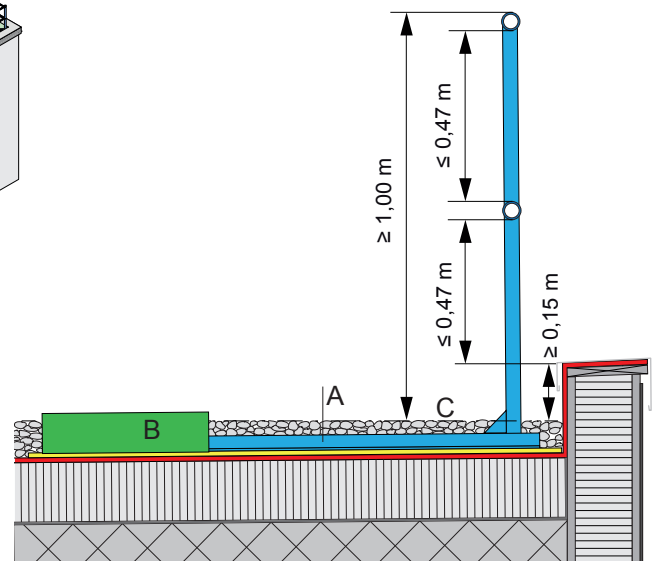
Fig. 17: Classe d'équipement 3: Système de protection latérale (A) avec le poids de retenue (B) sur le revêtement du toit plat, cotes depuis la couche d'usure/de protection (C)
