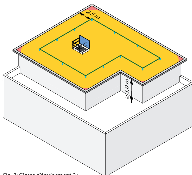
Fig. 7: Classe d'équipement 2 : Utiliser impérativement un système de retenue avec petit espace de chute, p. ex. avec des terrasses en attique ou des annexes avec des hauteurs moins de 6,25 m
