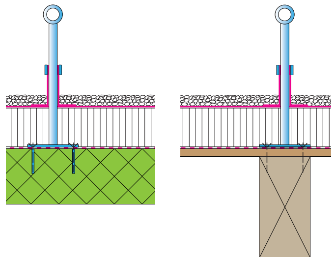
Fig. 3: Classe d'équipement 1 : PAI monté sur un toit plat avec isolation thermique, variante sur une charpente et sur du béton
