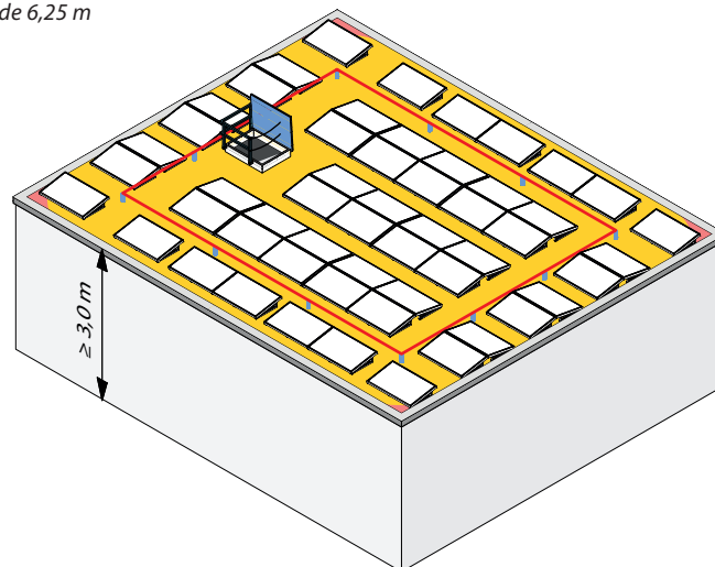
Fig. 8: Classe d'équipement 2 : Système de retenue avec des installations solaires couvrant toute la surface
