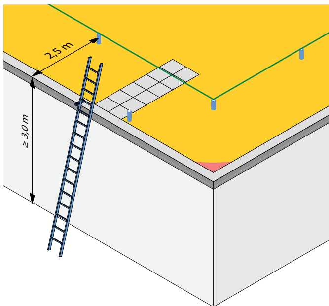
Fig. 19: Accès par une échelle simple, acceptable jusqu'à deux étages
