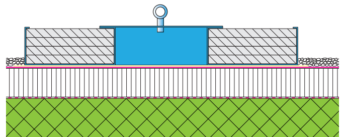
Fig. 4: Classe d'équipement 1 : Points d'ancrage avec le poids de retenue, sans perforation de l'étanchéité. Ces points peuvent être utilisés temporairement, mais pas lors de températures glaciales, p. ex. pour le déblaiement de neige.
