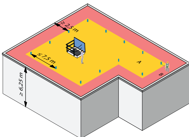
Fig. 2: Classe d'équipement 1: PAI adaptés au bord du toit en fonction de la géométrie du bâtiment
