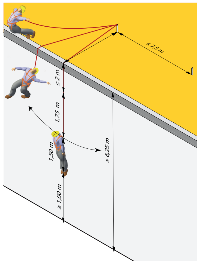
Fig. 11: Chute pendulaire sur un toit plat avec un espace de chute d'au moins 6,25 m
