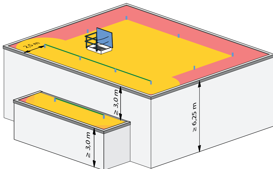
Fig. 12: Exemple avec terrasse en attique ou bâtiment avec annexe. Installation des classes d'équipement 1 et 2. Avec un espace de chute de moins de 6,25 m, la classe d'équipement 2 doit être exécutée. Exécution avec dispositif d'ancrage fixe ou temporaire.
