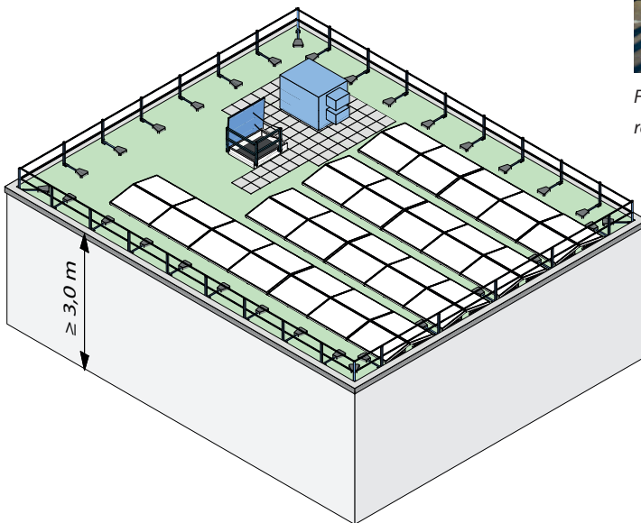
Fig. 15: Classe d'équipement 3 : Protection collective à recommander pour les toits plats auxquels on doit accéder plusieurs fois par année pour la maintenance ou d'autres travaux
