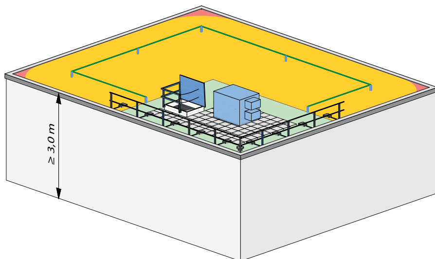
Fig. 13: Exemple de bâtiment industriel avec des climatiseurs sur la surface de toit. Installation des classes d'équipement 2 et 3. Avec des installations d'aération à maintenance intensive ou les travaux plus de 2 personnes/jours, ces zones de toit en classe d'équipement 3 sont à munir d'une protection latérale.
