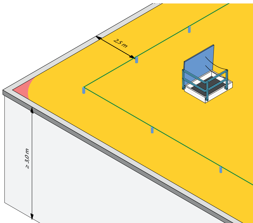
Fig. 21: Accès par un dispositif d'accès fixe. L'escalier d'accès doit être disposé de manière à ce que l'accès au toit se trouve dans la zone de danger intérieure
