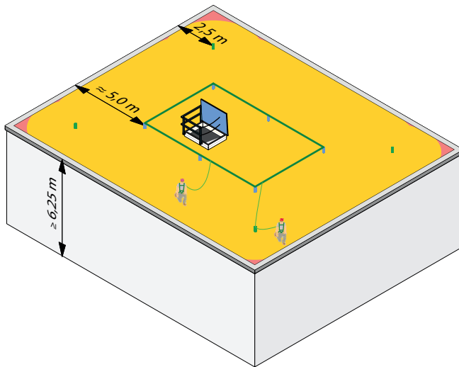
Fig. 9: Classe d'équipement 2 : Un système d'arrêt de chute combiné avec des PAI dans les coins
