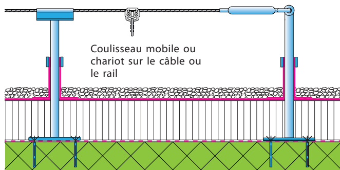
Fig. 5: Classe d'équipement 2 : le système à câble horizontal permanent avec tendeur, ancré dans le béton armé
