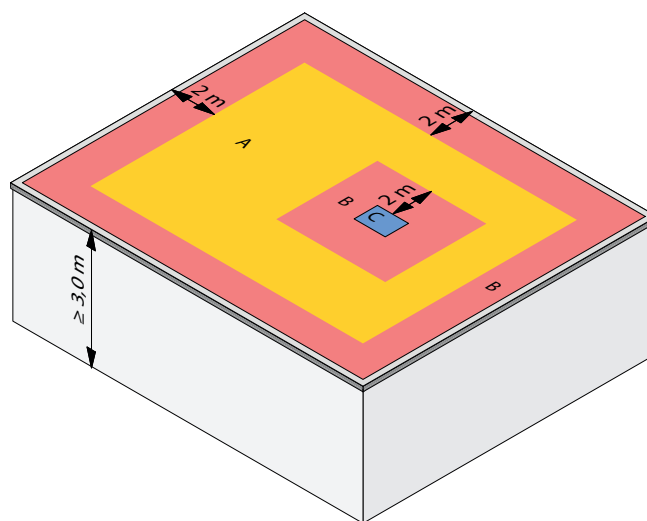
Fig. 1: (A) Zone de danger, (B) zone de danger particulier, (C) Coupole de toit avec zone de danger particulier ou avec une grille résistante à la rupture. La largeur de la zone de danger particulier est d'au moins 2 m, mesuré parallèlement au bord de chute.
