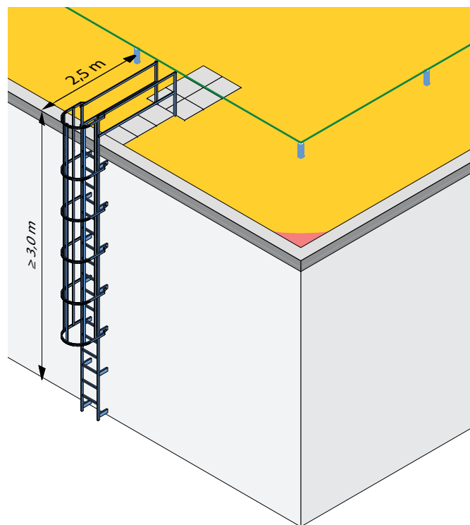
Fig. 20: Accès par une échelle fixe
